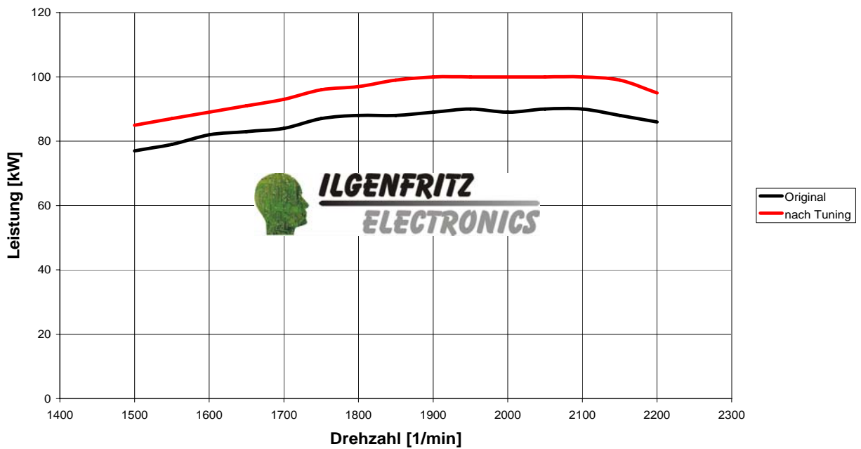
Drehzahl / Leistungskennlinie an der Zapfwelle gemessen
